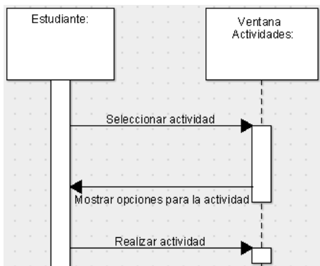
Figura 3. Ejemplo de un diagrama de secuencia. (Software Lenguaje Maya - Edupmedia-2008)
