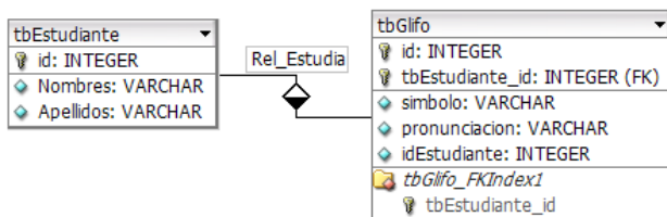
Figura 4. Vista parcial de un MER. (Software Lenguaje Maya - Edupmedia-2008 [10])
